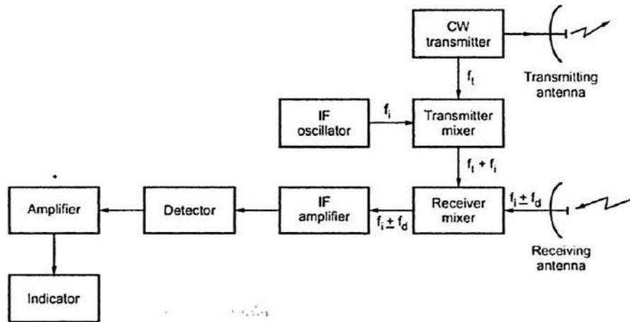
Fig. CW Doppler radar
